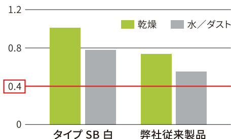
すべり抵抗係数／CSR'
